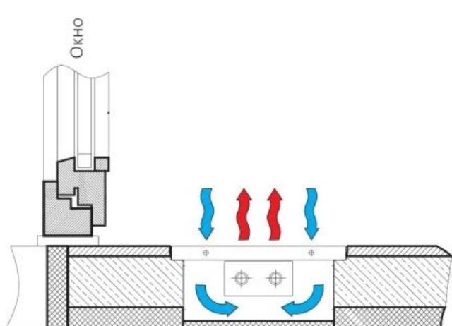
Естественная конвекция, KB3
