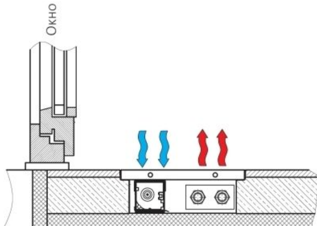
Принудительная конвекция, KB3B
